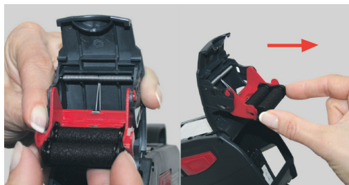
Kép 13 A festékhenger kivétele
