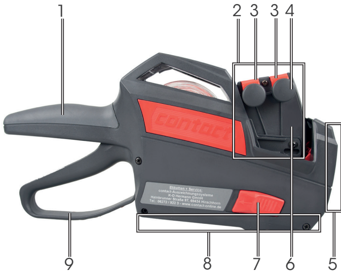
Kuva 1 Suljettu käsihinnoittelija – Näkymä sivulta
