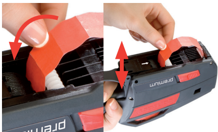
Figura 21 Papel de suporte entre o rolo inversor e a roda de transporte
