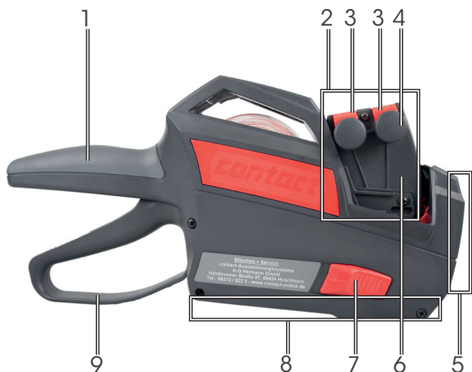
Figura 1 Etiquetadora manual fechada - vista lateral
