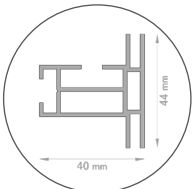
Aluminiumprofil 44 mm geschlossen:
