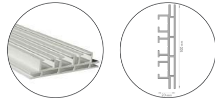
Einseitige und doppelseitige Ausleuchtung
