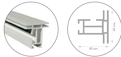
Aluminiumprofil 44 mm geschlossen:
