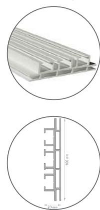
Aluminiumprofil 100 mm:
